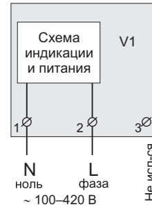
Схема 1. Упрощенная внутренняя схема и схема подключения
