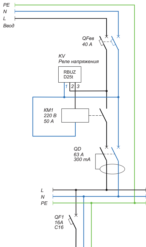
Схема 3. Вариант электрической схемы подключения реле RBUZ D25t и контактора с обмоткой 230 В
