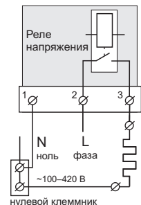
Схема 1. Упрощенная внутренняя схема и схема подключения
